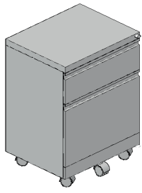
ARCHIVADOR 1x1 Ancho=64,5CM Alto=53,5CM Prof=45CM
